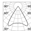
CRI≥80 40W 60° 5300lm 3000K
